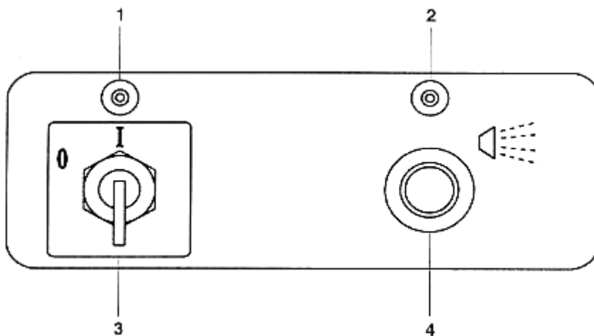
Рис.5 Блок управления
