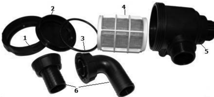
Рис. 5. Фильтр всасывающий.
