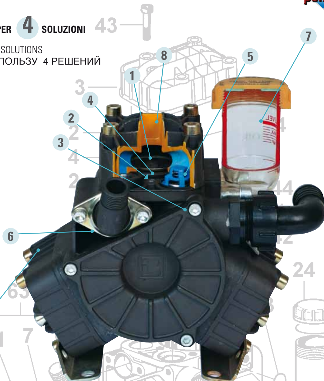
CARATTERISTICHE COSTRUTTIVE POMPE PA - PA PUMPS MANUFACTURING FEATURES КОНСТРУКТИВНЫЕ ХАРАКТЕРИСТИКИ НАСОСОВ PA
